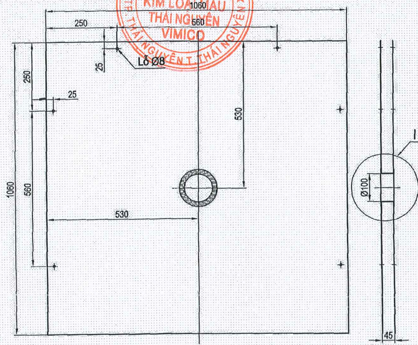
TỦI VÀI LỌC ÉP LOẠI 1,06m x 1,06m
