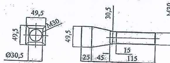
BU LÔNG BẮT TÂM LÓT THÂN TANG
