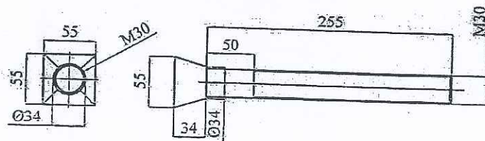
BU LÔNG BẮT TÂM LÓT CANH LOẠI 2
