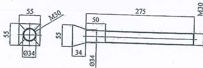
BU LÔNG BẮT TÂM LÓT CANH LOẠI 1
