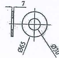
GIOĂNG ĐEM KÍN BU LÔNG
